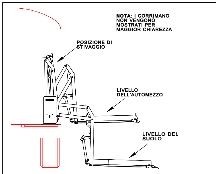
FIGURA 4: POSIZIONI DELLA PIATTAFORMA
